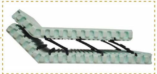
מבט על רשת מתקפלת בעלת צירים מתכתיים, ורשת תוסף לפינות זוויתיות (בכללת בהזמנה).
